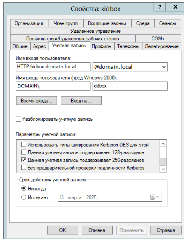
Рисунок 1 – Настройка учетной записи в Active Directory
